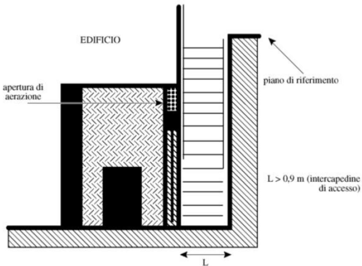
Tavola 2b - Locale interrato
