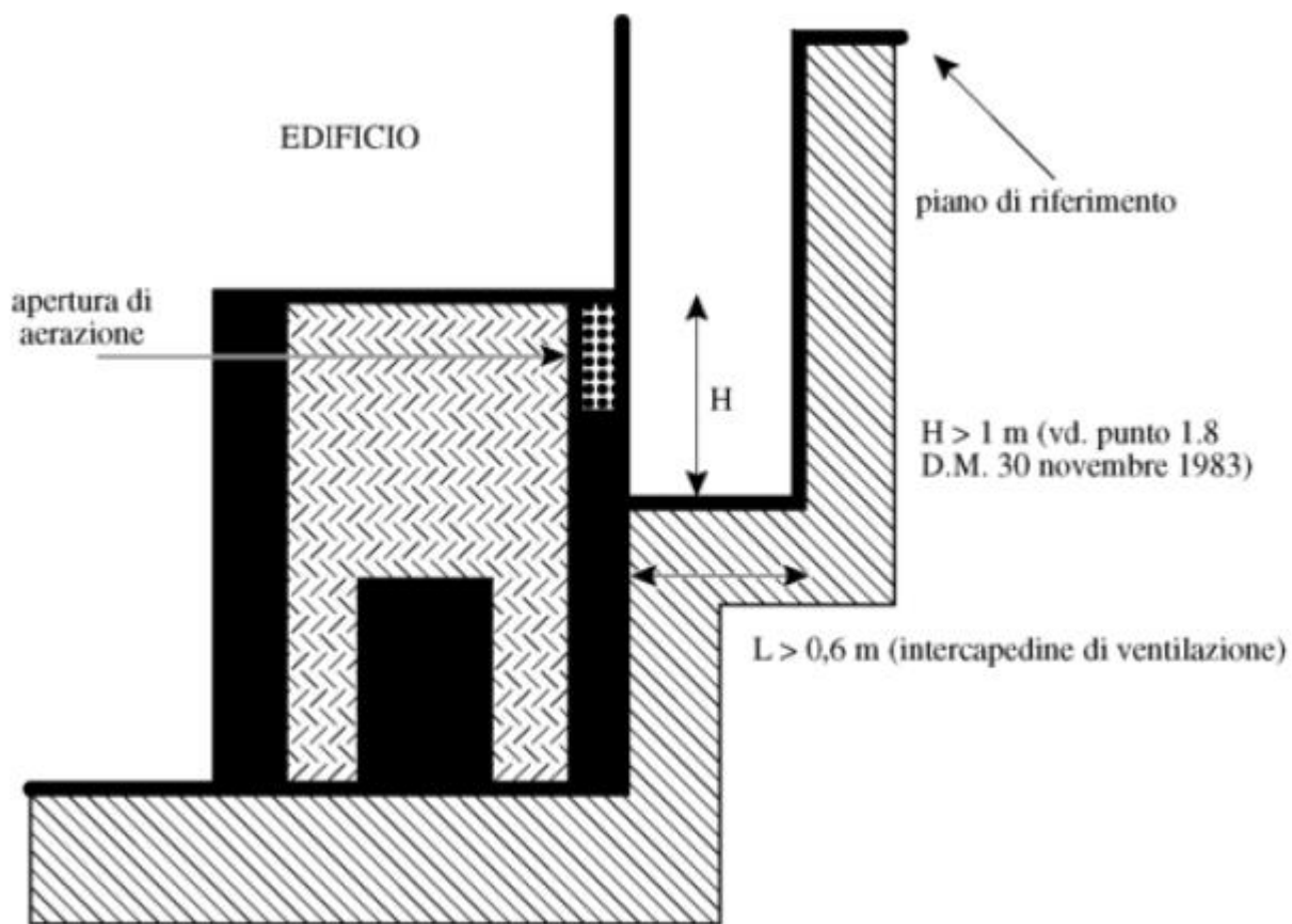
Tavola 2b - Locale interrato
