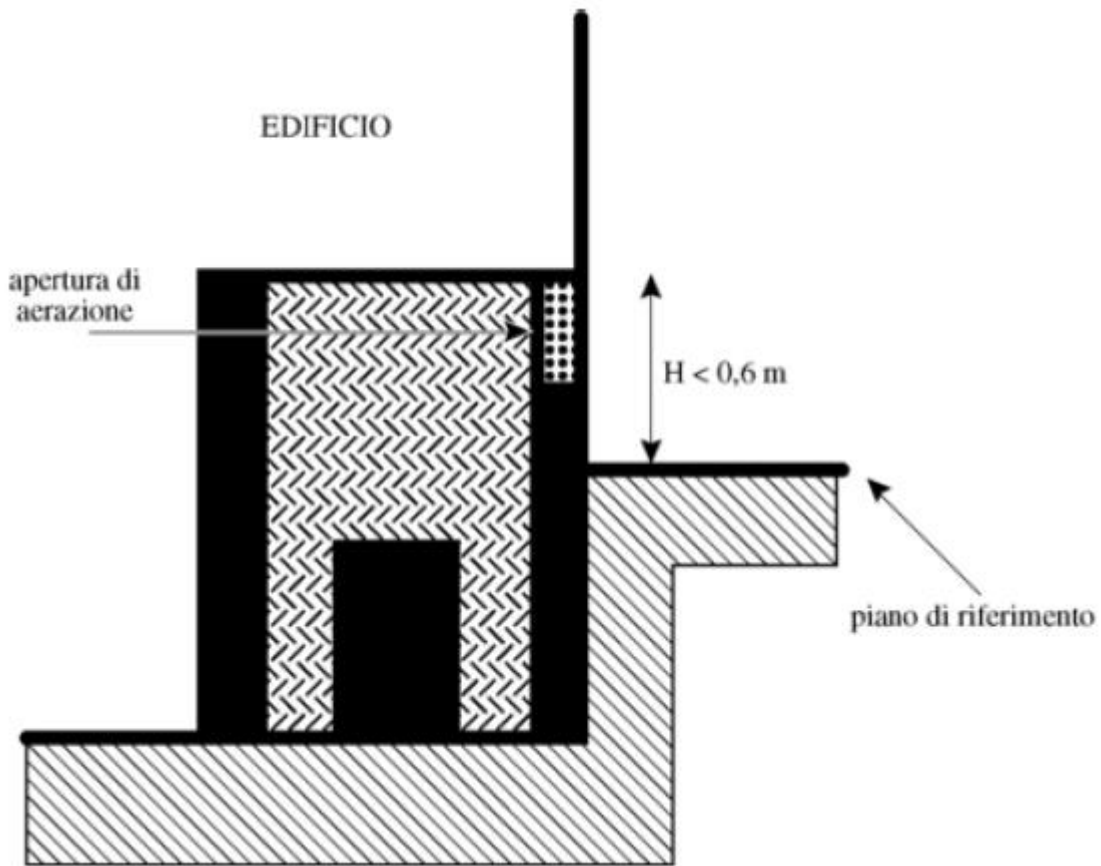
Tavola 2c - Locale interrato
