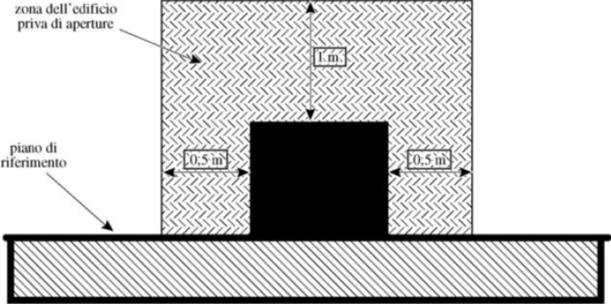
Tavola 4 - Installazione all'aperto in adiacenza a parete
