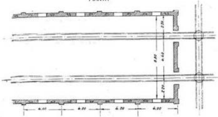
TIPO DI BARACCA PER MATERIALI ESPLOSIVI PIANTA
